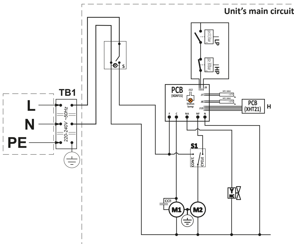
Wiring diagram DH 20
